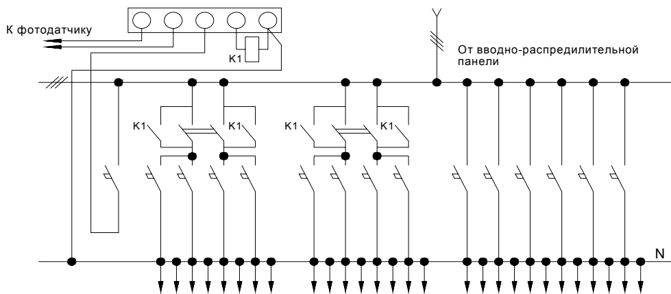
Рис.5.21 (Схема БОУ-43).
