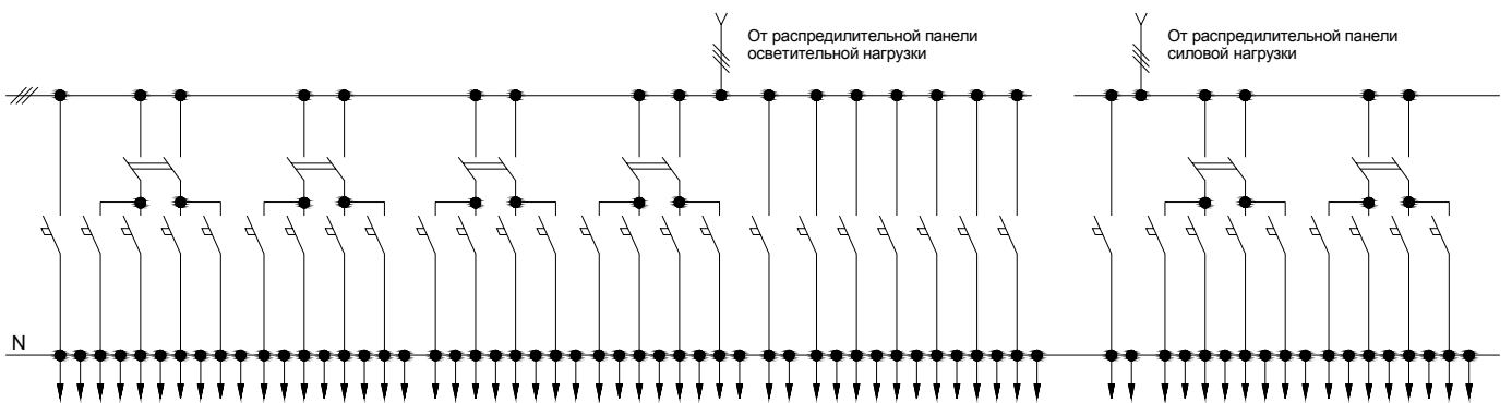
Рис.5.26 (Схема БОУ-02).
