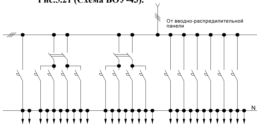
Рис.5.22 (Схема БОУ-44).
