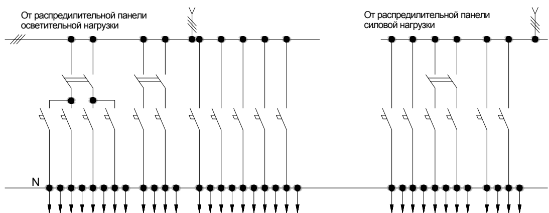
Рис.5.28 (Схема БОУ-04).
