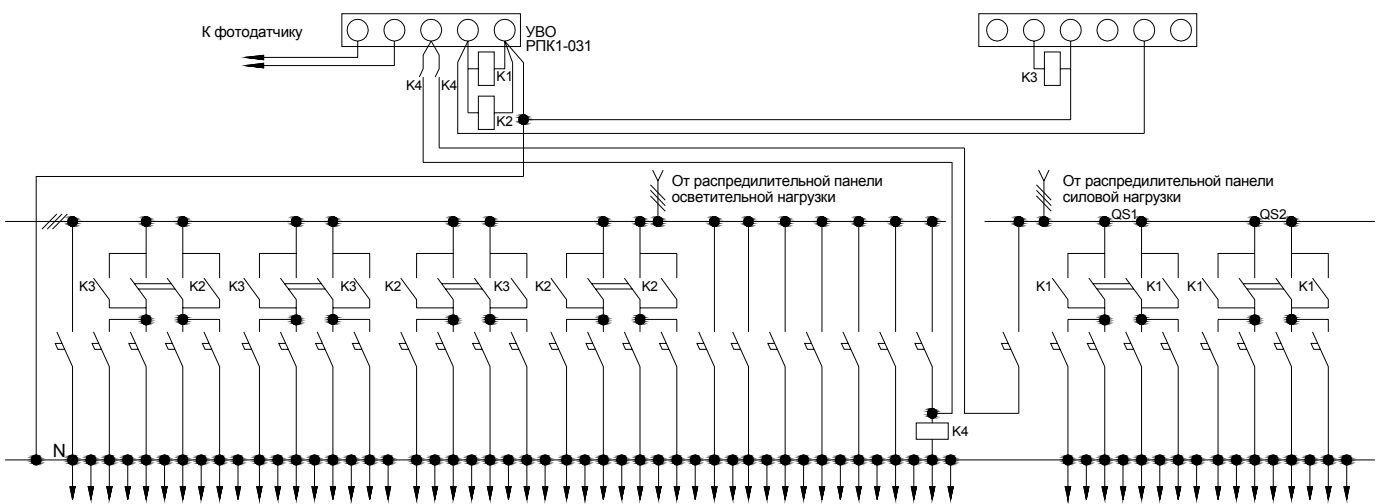
Рис.5.25 (Схема БОУ-01).
