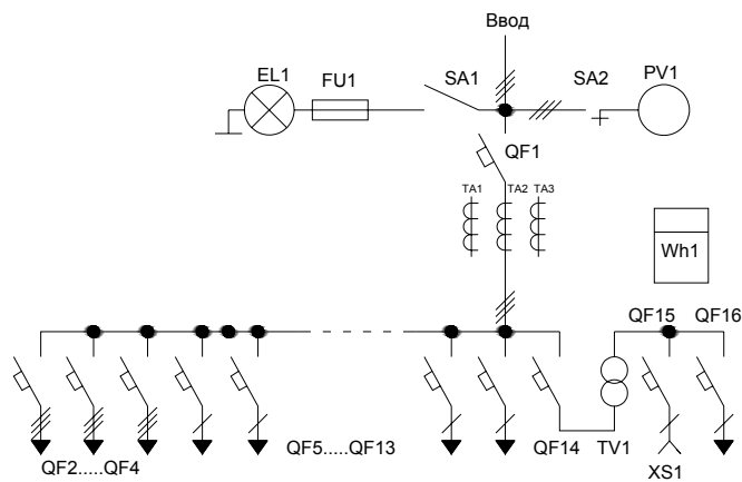
Рис.6.9 Устройство вводно-распределительное ЯВР 95-2.
