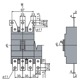
Разметка монтажных отверстий
