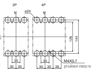
Разметка монтажных отверстий
