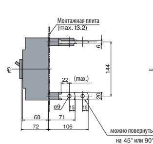
Заднее подключение
