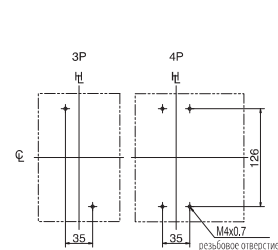
Разметка монтажных отверстий
