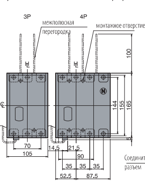
Заднее подключение
