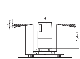
Положение петель (защитная область) вид снизу
