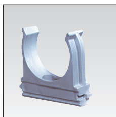
Держатель труб с защелкой Производитель - Elettrocanali (Италия) Материал - самопотухающий ПВХ Цвет - серый RAL 7035
