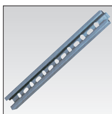
Рейка для держателей труб Производитель - Elettrocanali - L.A.P. Srl (Италия) Материал - самопотухающий ПВХ Цвет - серый RAL 7035
