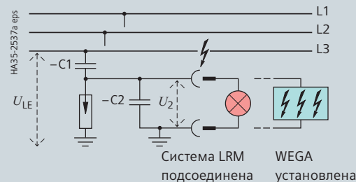
Индикация напряжения через емкостной делитель напряжения (принципиальная схема)
