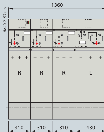
Схема RRRL
