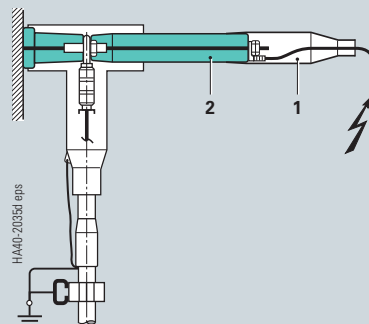
Испытание кабеля в месте расположения кабельного T-образного адаптера (Пример)
