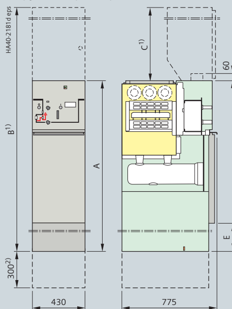
Продольная разъединительная ячейка сборной шины, тип Н с комбинированным выключателем нагрузки с предохранителем
