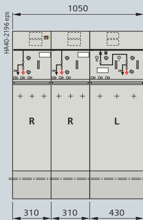
Схема RRL
