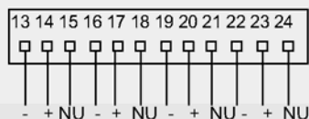
Импульсный ввод – слоты с A до F (Положение коннектора справа)
