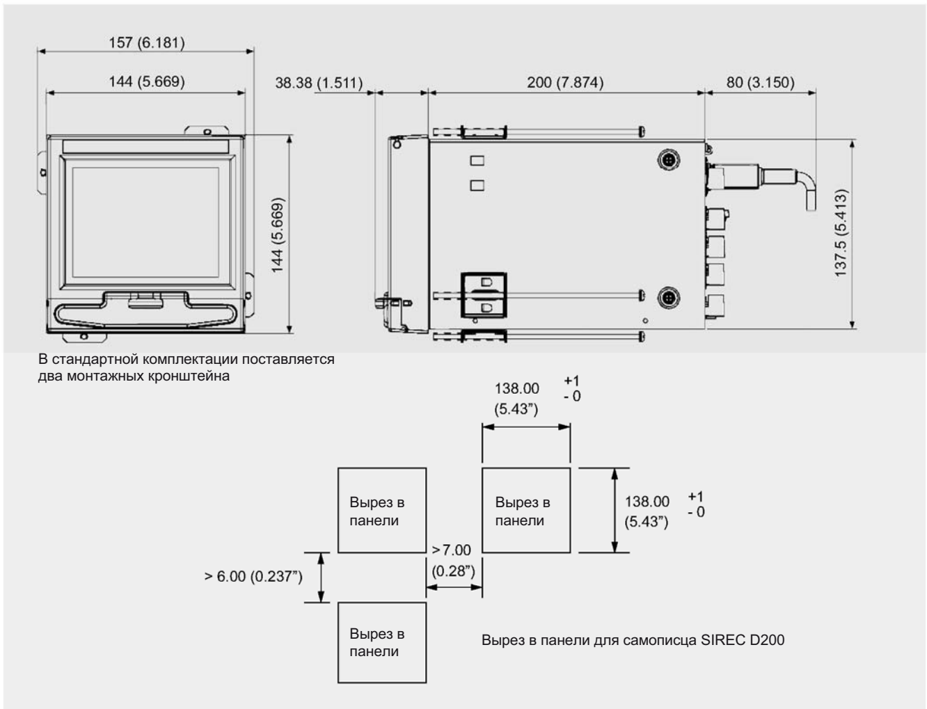
SIREC D200, размеры в мм (дюймах) и вырез в панели
