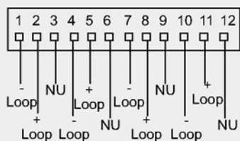
Импульсный ввод – слоты с A до F (Положение коннектора справа)
