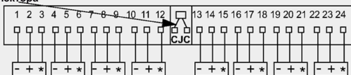
СJC Положение коннектора
