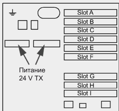
Аналоговый вывод – слоты E и F
