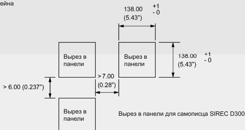
SIREC D300, размеры в мм (дюймах) и вырез в панели
