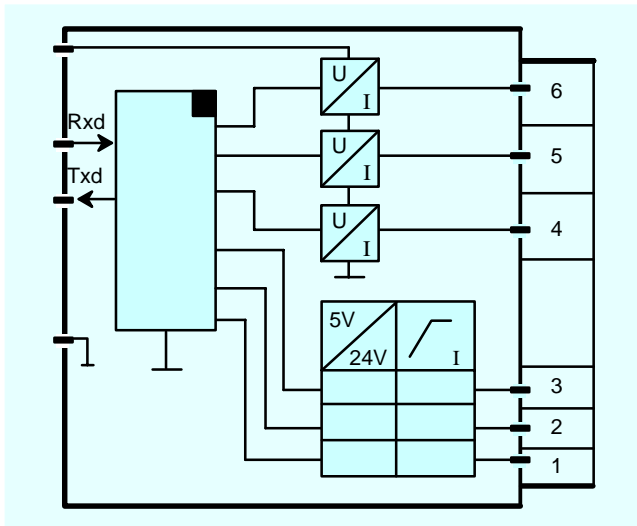
Fig. 6/17 Wiring of 3AO/3DI module
