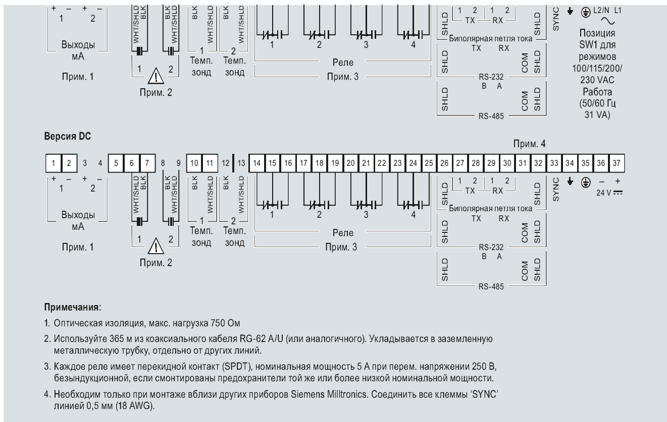
Соединения SITRANS LU01
