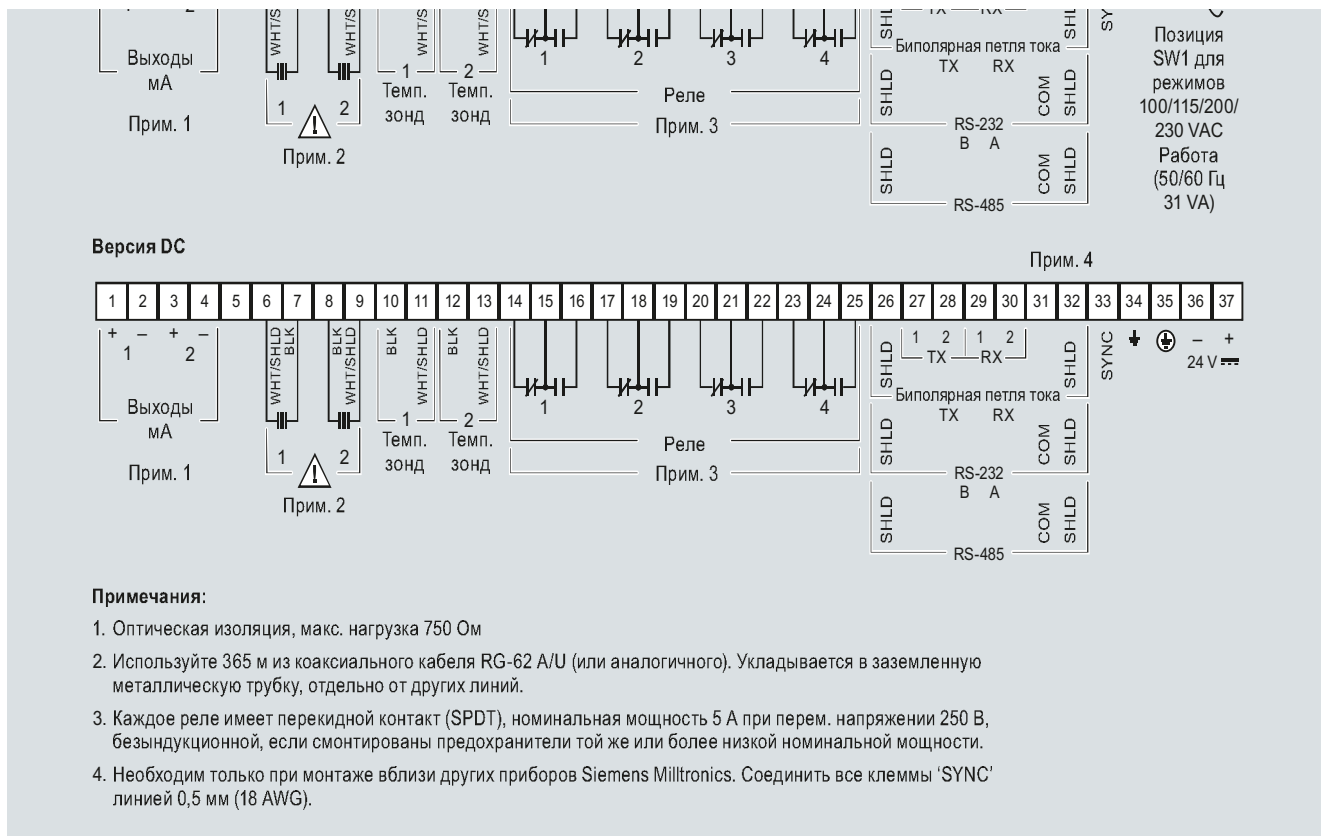
Соединения SITRANS LU02
